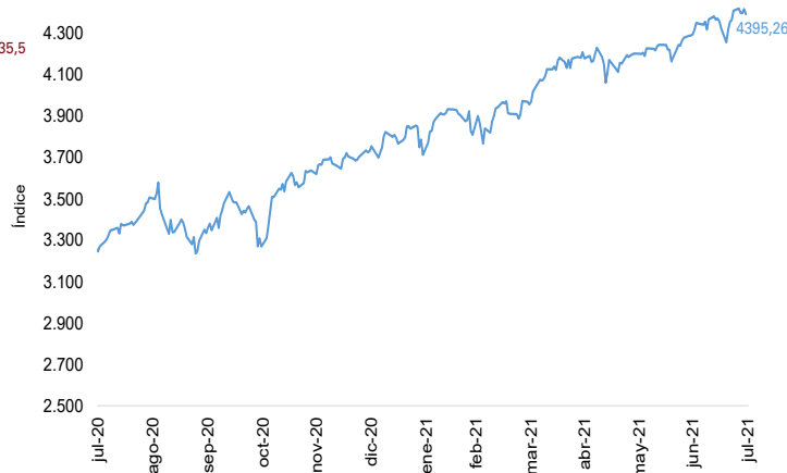
Índice S&P 500
