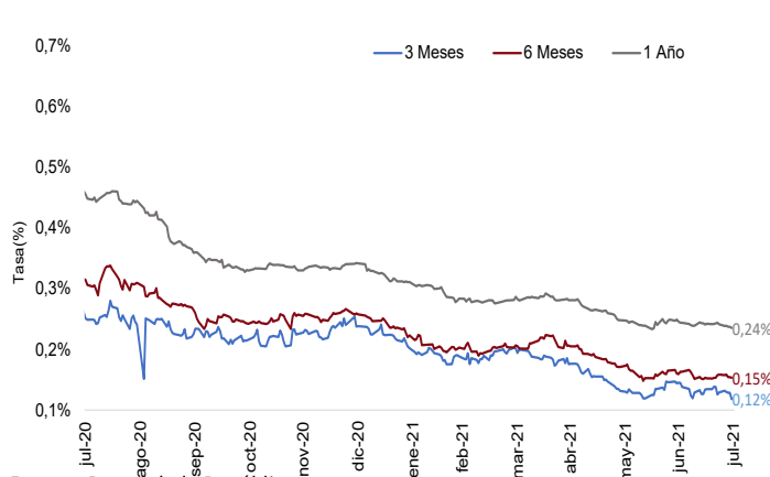
Tasa LIBOR
