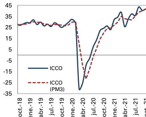
Gráfico 3. ICCO (Balance, %)
