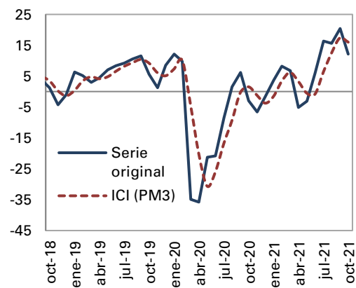
Gráfico 4. ICI (Balance, %)
